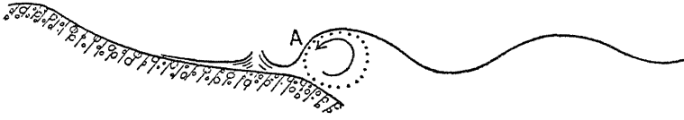
चित्र १२७—विनाशकारी तरंगों का टूटना।
